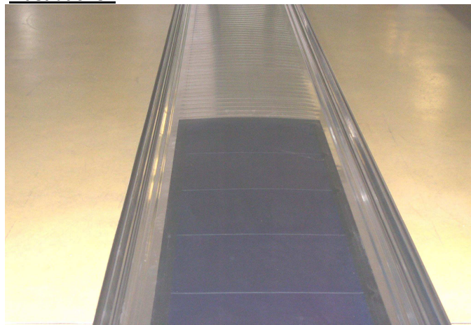
Photovoltaïque intégré sur profil
