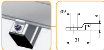
Équerre de fixation 10005
