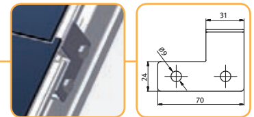
Butée d'extrémité S2plus 10003
